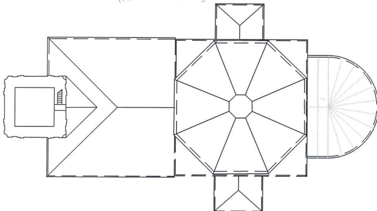
План - схема кровли (РЕКОНСТРУКЦИЯ)
