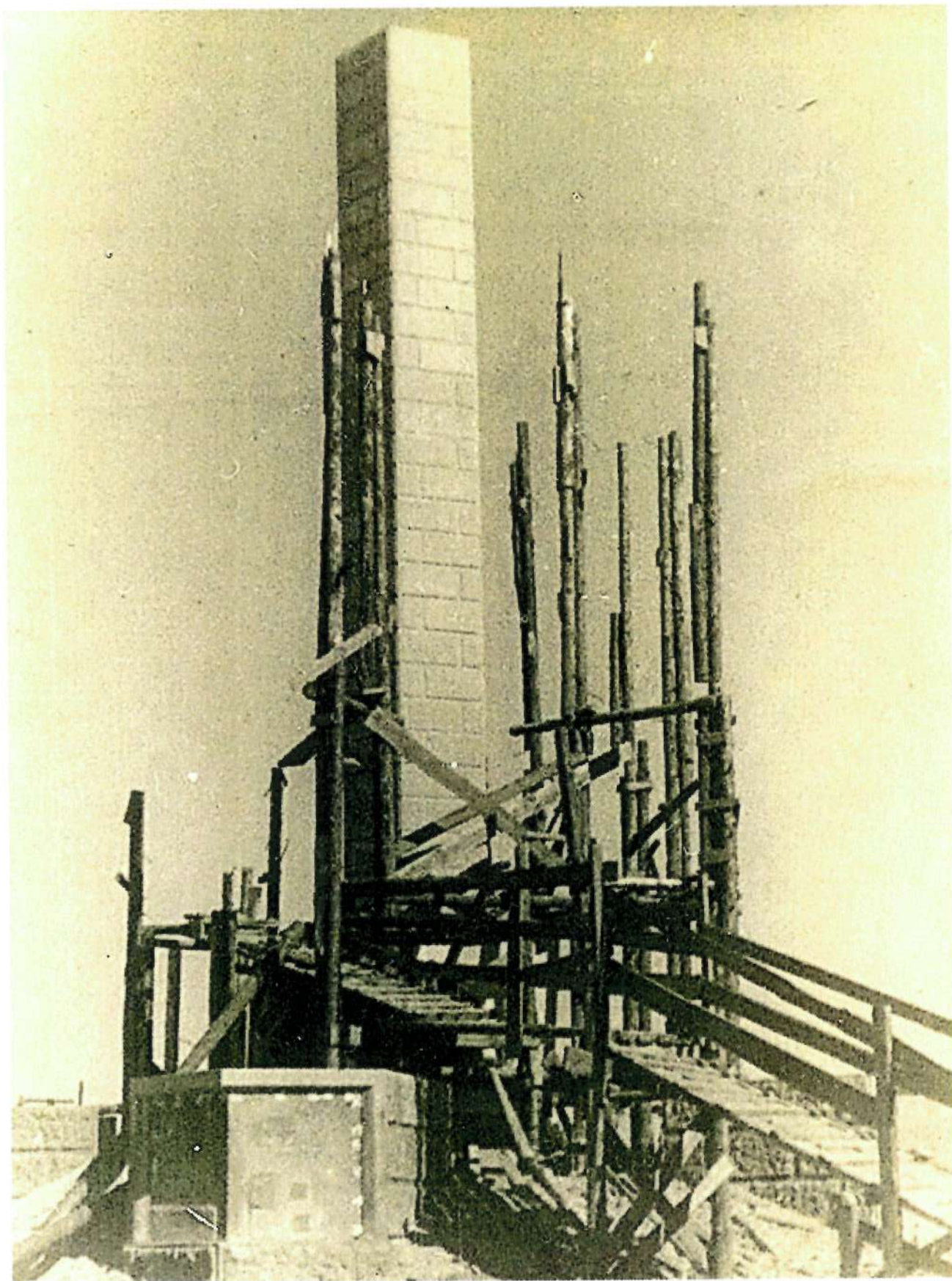
Разборка лесов по завершению строительства пилон памятника. 1947 г.
