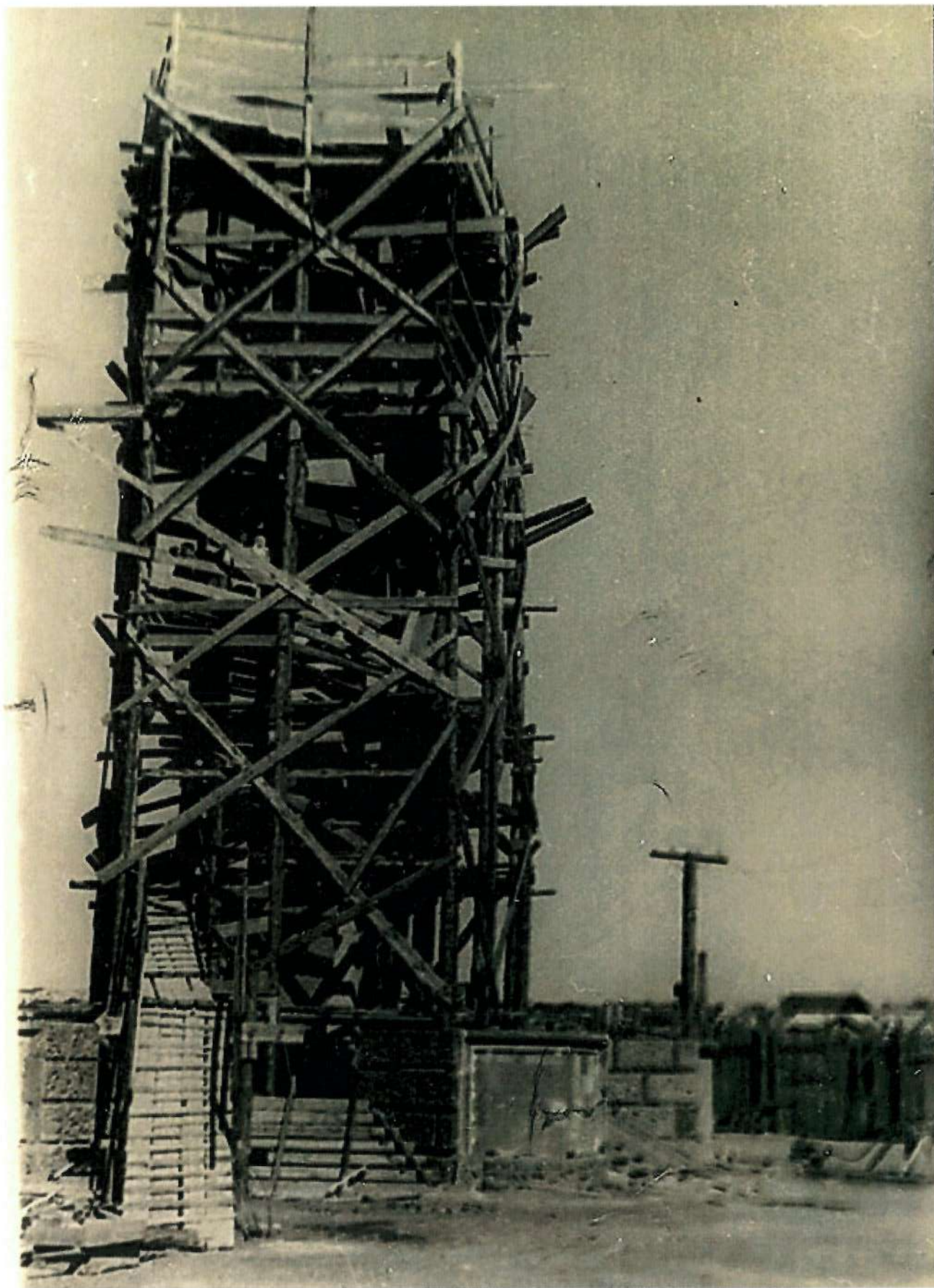
Начало строительства памятника. Устройство лесов для постройки пилона на сооруженном основании памятника. 1947 г.
