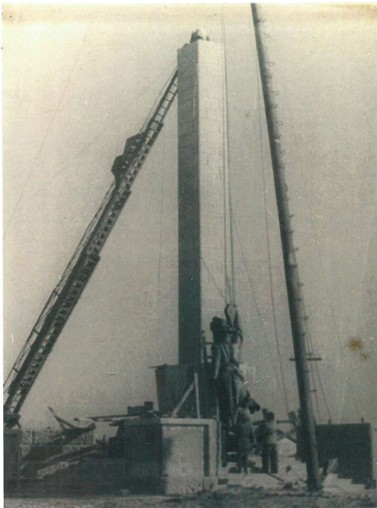
Подъем статуи на вершину пилона. 1947 г.
