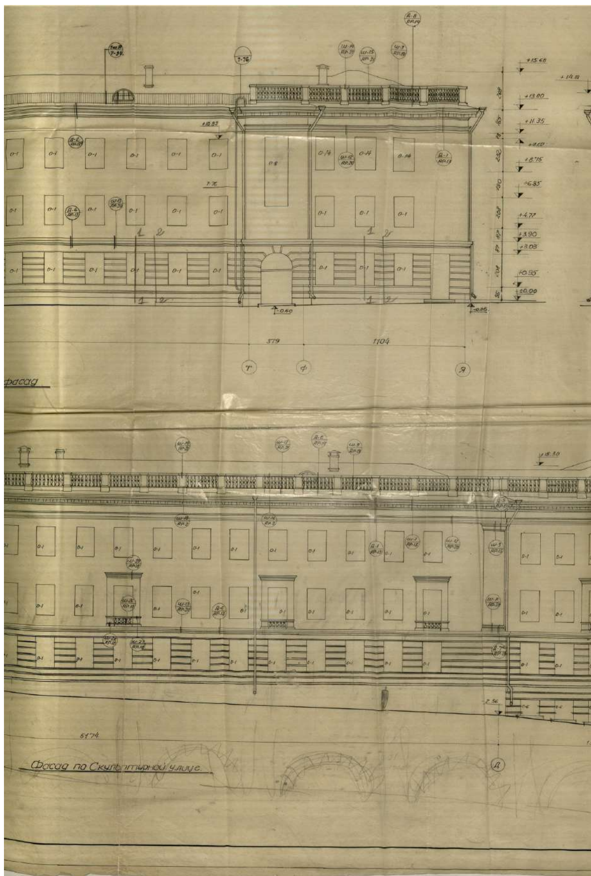
9. Чертеж «Заглавный лист проекта «Больница имени Ильича. Главный корпус. Вторая очередь строительства». Общий вид 2. Ф.Р-2, Оп. 5, Д.2, Л. 1 (фрагмент)
