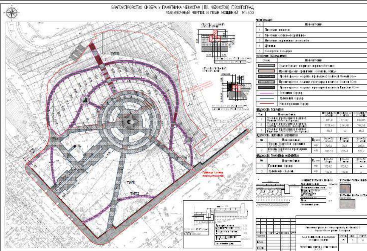
Разбивочный чертеж и план мощения
