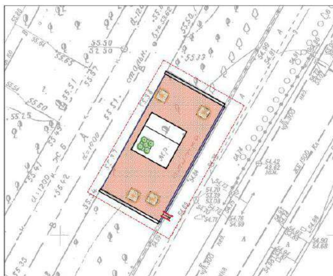
Схема 2 . Генеральный план участка благоустройства. М. 1:500.
