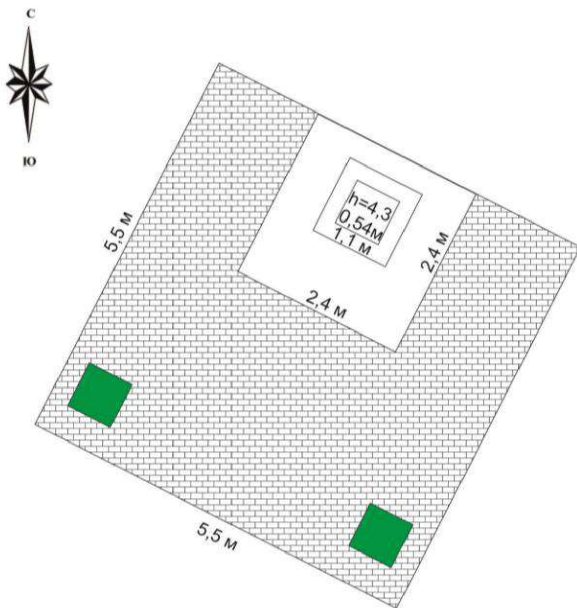
Схема локальных промеров.
